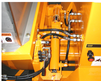
Люлеещ механизъм с два цилиндъра
